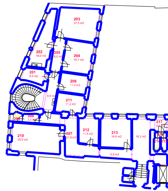
PŮDORYS 3NP
