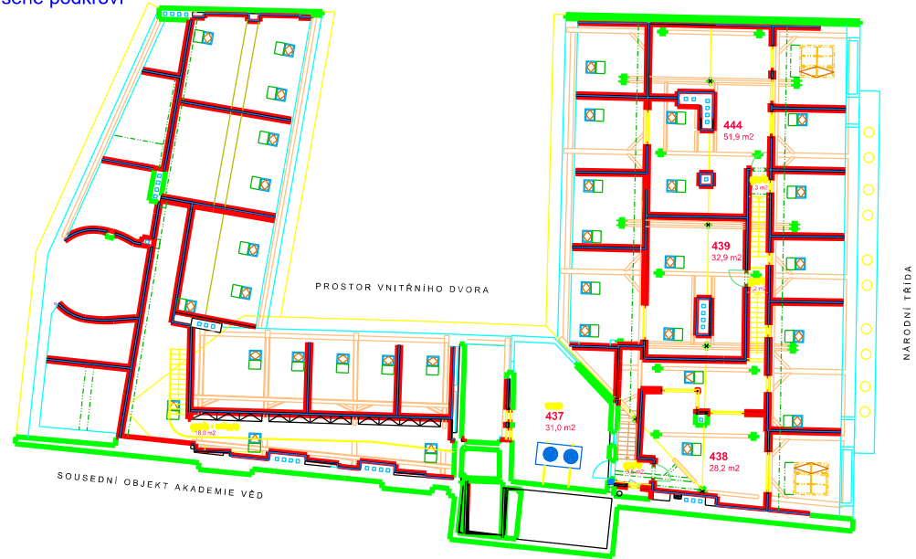
PŮDORYS 5NP zvýšené podkroví
