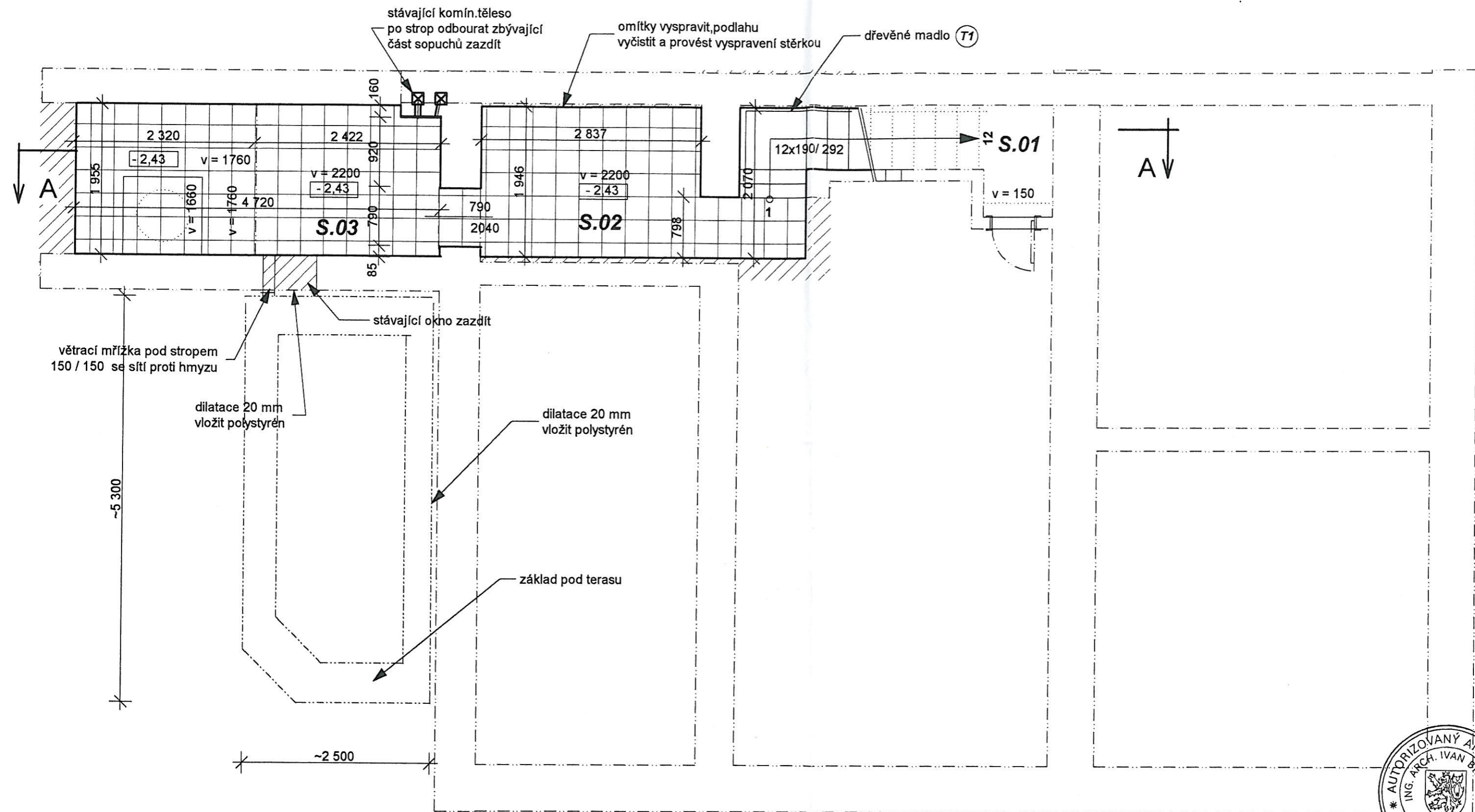
ZÁKLADY dle arch. dokumentace
